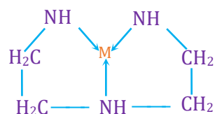
Diethylene triamine (Dien)
